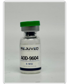
AOD-9604 5mg - AOD5-101
